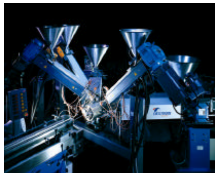
五层共挤挤出机组
